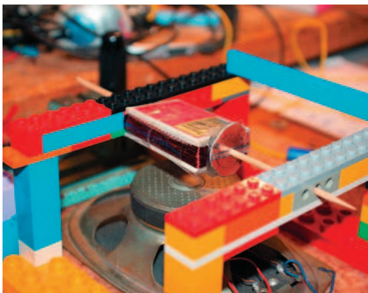
▲ Vít Nožka, konstrukce jednoduchého elektromotoru
